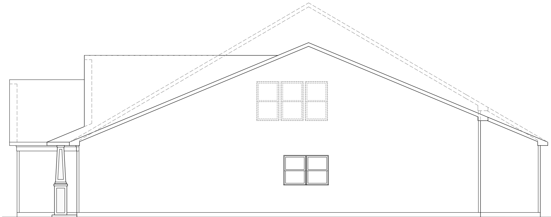
RIGHT ELEVATION
